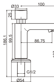
T05 Grifo para lavabo Temporizado Time delay wash basin tap Robinet temporisé
