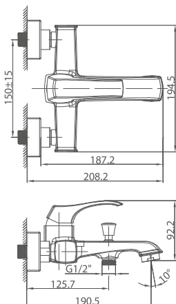
JED1463C Monomando para baño/ducha Bath/shower mixer Mitigeur de bain/douche
