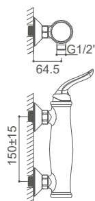
DXB1074C Monomando para ducha Shower mixer Mitigeur de douche
