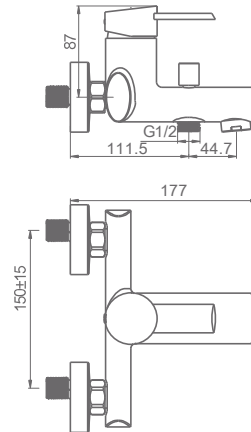
FRA1273C Monomando para baño/ducha Bath/shower mixer Mitigeur de bain/douche
