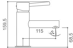
MIL0341C Monomando para lavabo Wash basin mixer Mitigeur de lavabo
