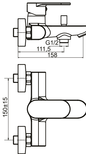
ATL1263C Monomando para baño/ducha Bath/shower mixer Mitigeur de bain/douche
