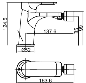
GIR2542C Monomando para bidé Bidet mixer Mitigeur de bidet
