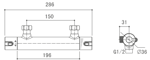
DFW09C COOL TOUCH Termostático para ducha Shower thermostatic mixer Mitigeur thermostatique de douche
