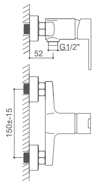
ORD0234C Monomando para ducha Shower mixer Mitigeur de douche
