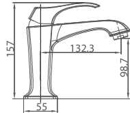
JED1461C Monomando para lavabo Wash basin mixer Mitigeur de lavabo
