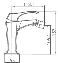
JED1462C Monomando para bidé Bidet mixer Mitigeur de bidet
