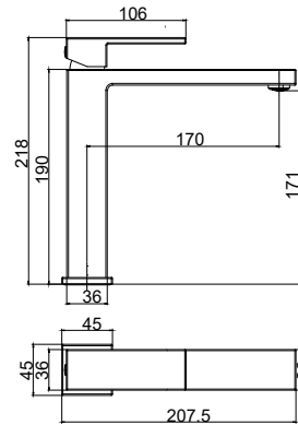
CAT1711-2C Monomando para lavabo ALTO Wash basin mixer HIGH Mitigeur de lavabo HAUT
