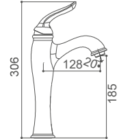
DXB10711C Monomando para lavabo ALTO Wash basin mixer HIGH Mitigeur de lavabo HAUT
