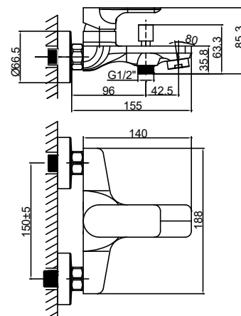
GIR2543C Monomando para baño/ducha Bath/shower mixer Mitigeur de bain/douche
