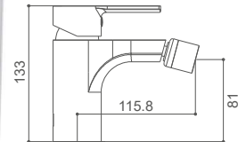
ROM0562CB Monomando para bidé Bidet mixer Mitigeur de bidet
