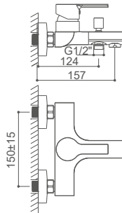
ROM0563CV Monomando para baño Bath mixer Mitigeur de bain
