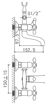
SAF6003C Grupo para baño Bath mixer Melangeur de bain
