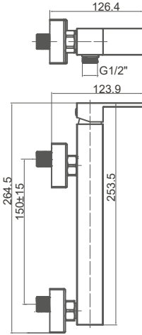
CAT1714C Monomando para ducha Shower mixer Mitigeur de douche
