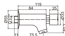
T06 Grifo pared Temporizado Time delay wall tap Robinet temporisé
