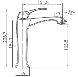
JED14611C Monomando para lavabo MEDIO Wash basin mixer MEDIUM Mitigeur de lavabo MOYEN
