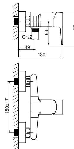
JFK2294C Monomando para ducha Shower mixer Mitigeur de douche
