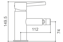
MIL0342C Monomando para bidé Bidet mixer Mitigeur de bidet
