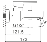
LHR3903C Monomando para baño/ducha Bath/shower mixer Mitigeur de bain/douche
