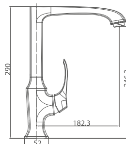
JED1465C Monomando para cocina Kitchen mixer Mitigeur de cuisine
