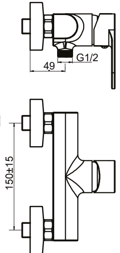
ATL1264C Monomando para ducha Shower mixer Mitigeur de douche
