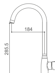
ROM0565CB Monomando para cocina Kitchen mixer Mitigeur de cuisine
