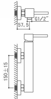
AMS9204C Monomando para ducha Shower mixer Mitigeur de douche
