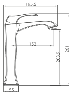
JED14612C Monomando para lavabo ALTO Wash basin mixer HIGH Mitigeur de lavabo HAUT
