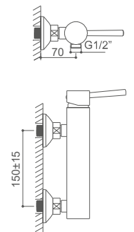
MIL0344C Monomando para ducha Shower mixer Mitigeur de douche
