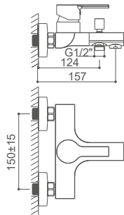
ROM0563CB Monomando para baño Bath mixer Mitigeur de bain
