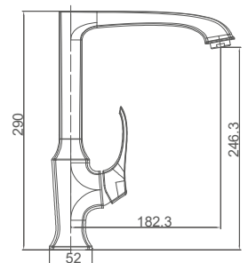
JED1465C Monomando para cocina Kitchen mixer Mitigeur de cuisine
