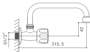
07733-AC Monobloc para cocina pared Wall Kitchen mixer Melangeur de cuisine
