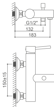
MIL0343C Monomando para baño/ducha Bath/shower mixer Mitigeur de bain/douche
