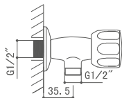
07010C Llave esquadra Angle valve Robinet d'equerre
