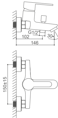
ORD0233C Monomando para baño/ducha Bath/shower mixer Mitigeur de bain/douche
