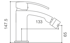
LAX0482C Monomando para bidé Bidet mixer Mitigeur de bidet
