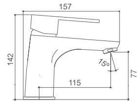
ORD02311C Monomando para lavabo MAXI Wash basin mixer MAXI Mitigeur de lavabo MAXI
