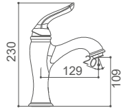
DXB1071C Monomando para lavabo Wash basin mixer Mitigeur de lavabo
