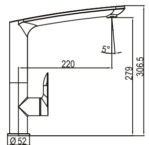
RIO2325C Monomando para cocina Kitchen mixer Mitigeur de cuisine
