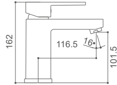
LHR3901C Monomando para lavabo Wash basin mixer Mitigeur de lavabo
