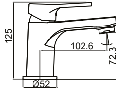
LIS2551C Monomando para lavabo Wash basin mixer Mitigeur de lavabo
