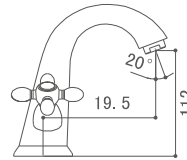
SAF60011C Monobloc para lavabo ALTO Wash basin mixer HIGH Melangeur de lavabo HAUT
