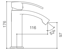
LAX0481C Monomando para lavabo Wash basin mixer Mitigeur de lavabo
