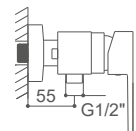
LHR3904C Monomando para ducha Shower mixer Mitigeur de douche
