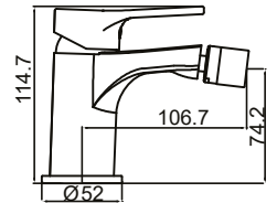
LIS2552C Monomando para bidé Bidet mixer Mitigeur de bidet
