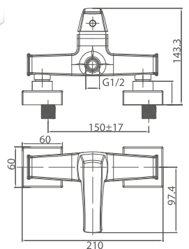
JED1464C Monomando para ducha Shower mixer Mitigeur de douche
