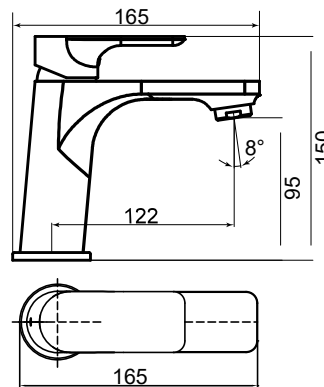
GIR25411C Monomando para lavabo ALTO Wash basin mixer HIGH Mitigeur de lavabo AUT
