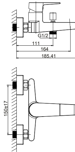
JFK2293C Monomando para baño/ducha Bath/shower mixer Mitigeur de bain/douche
