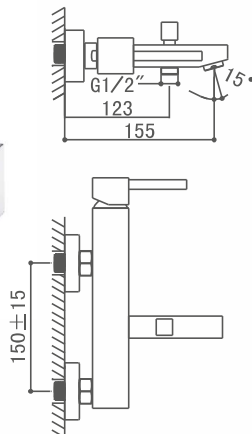
AMS9203C Monomando para baño/ducha Bath/shower mixer Mitigeur de bain/douche
