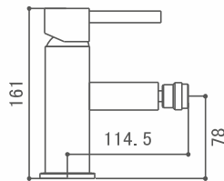
AMS9202C Monomando para bidé Bidet mixer Mitigeur de bidet
