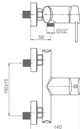
FRA1274C Monomando para ducha Shower mixer Mitigeur de douche
