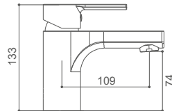
ROM0561CB Monomando para lavabo Wash basin mixer Mitigeur de lavabo
