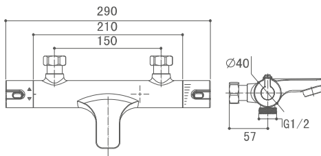
DFW08C COOL TOUCH Termostático para baño/ducha Bath/shower thermostatic mixer Mitigeur thermostatique de bain/douche
