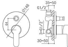
Monomando para baño/ducha Bath/shower mixer Mitigeur de bain/douche
