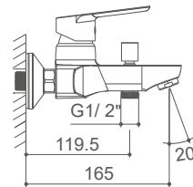
PEK0763C Monomando para baño/ducha Bath/shower mixer Mitigeur de bain/douche
