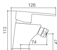
ORD0232C Monomando para bidé Bidet mixer Mitigeur de bidet
