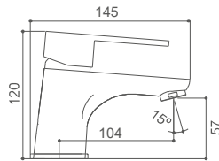
ORD0231C Monomando para lavabo Wash basin mixer Mitigeur de lavabo
