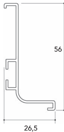
Soporte Fijación Metálico
