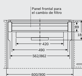
Diseño constructivo A Montaje en aparatos con bastidor de descenso - profundidad del cuerpo del mueble conforme a la tabla de combinaciones
