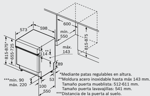
SMI46MS01E Dimensiones en mm
