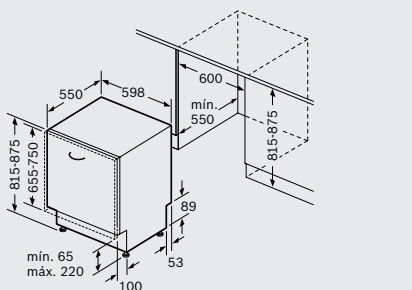
SME46MX03E Dimensiones en mm
