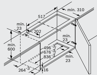
Montaje del componente del ventilador con módulo Clean Air
