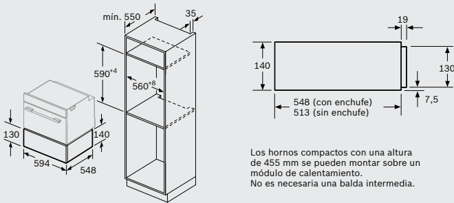
BIC630NS1, BIC630NW1, BIC630NB1
