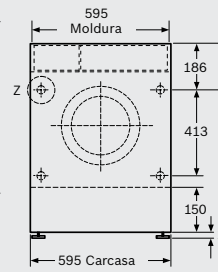
Dimensiones en mm
