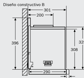
Diseño constructivo B Montaje en aparatos con bastidor (X) de descenso - profundidad del cuerpo del mueble conforme a la tabla de combinaciones
