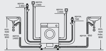
Dimensiones en mm
