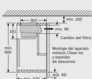
Montaje del componente del ventilador con módulo Clean Air
