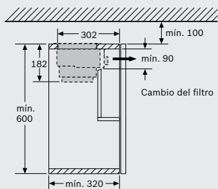
Montaje de la campana telescópica con módulo Clean Air
