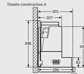
Diseño constructivo A Montaje en aparatos con bastidor de descenso - profundidad del cuerpo del mueble conforme a la tabla de combinaciones
